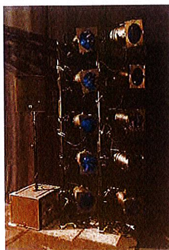
Vue côté cour – 2x plans PAR Cp62
